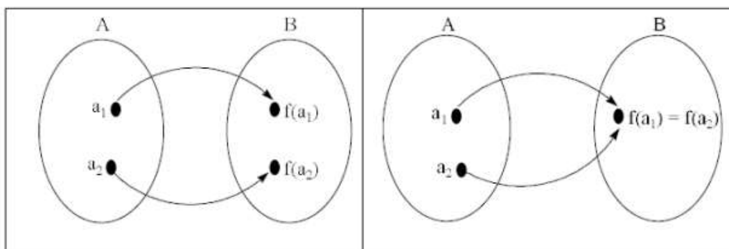
תרשים 1.4.2: מימין פונקציה שאינה חח"ע ומשמאל פונקציה חח"ע.
