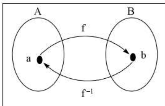
תרשים 1.4.5: הפונקציה f והפונקציה ההופכית ל- f .
